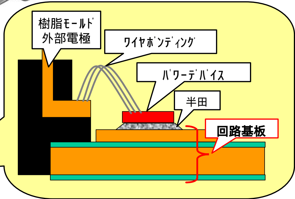
パワーモジュール内部構造
