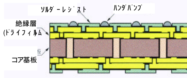
構造模式図
